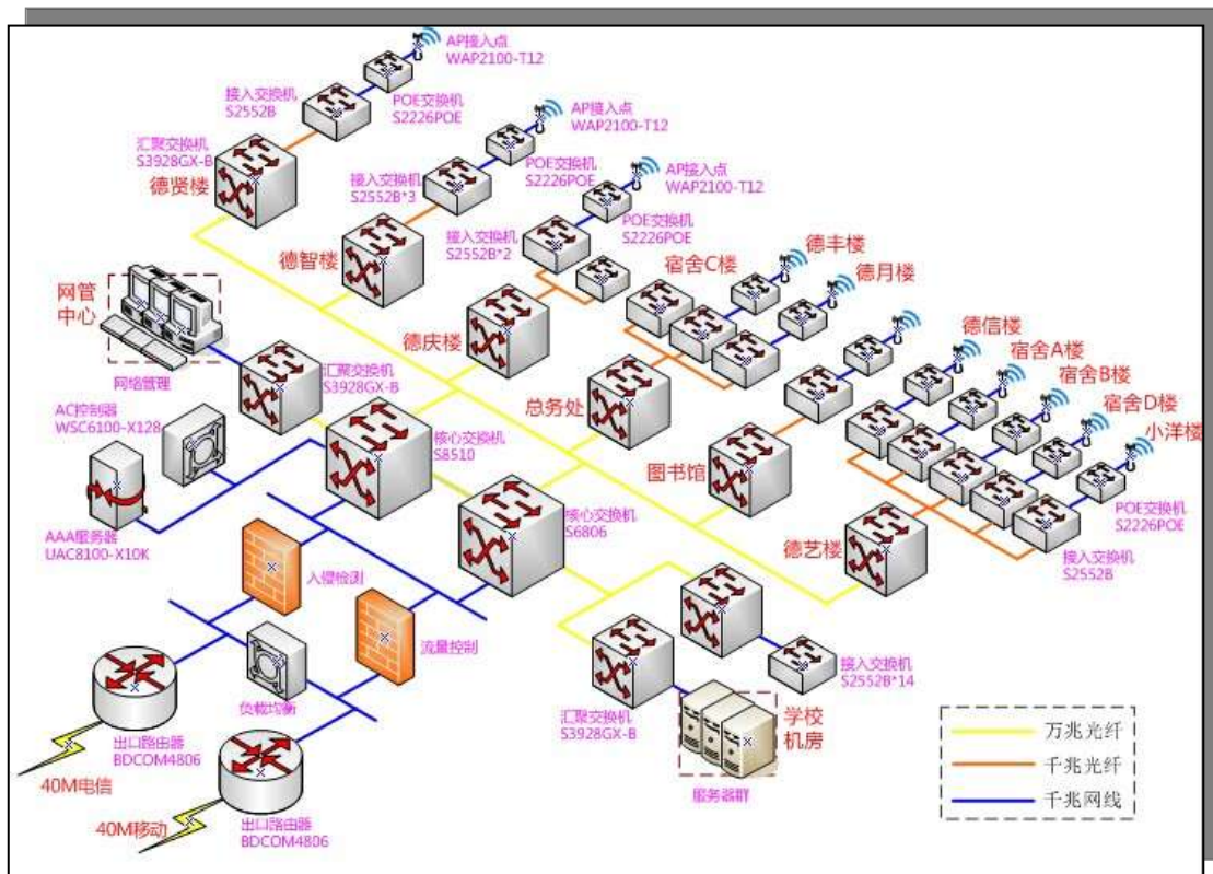
附图：邦德职业技术学院校园网络拓扑图
